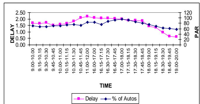
Figure 5.18: Delays vs. PAR
