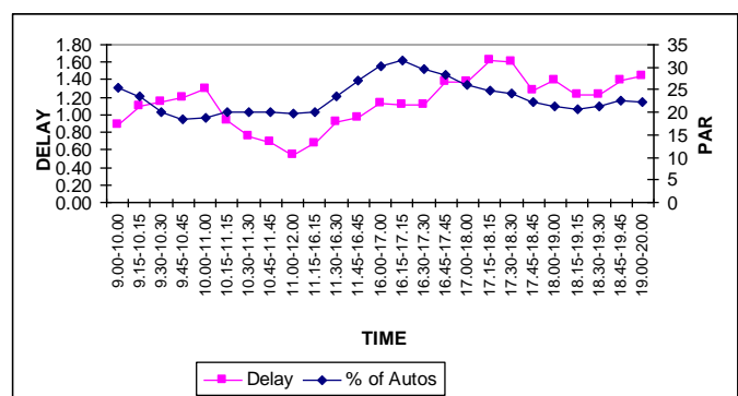
Figure 5.8: Delays vs. PAR
